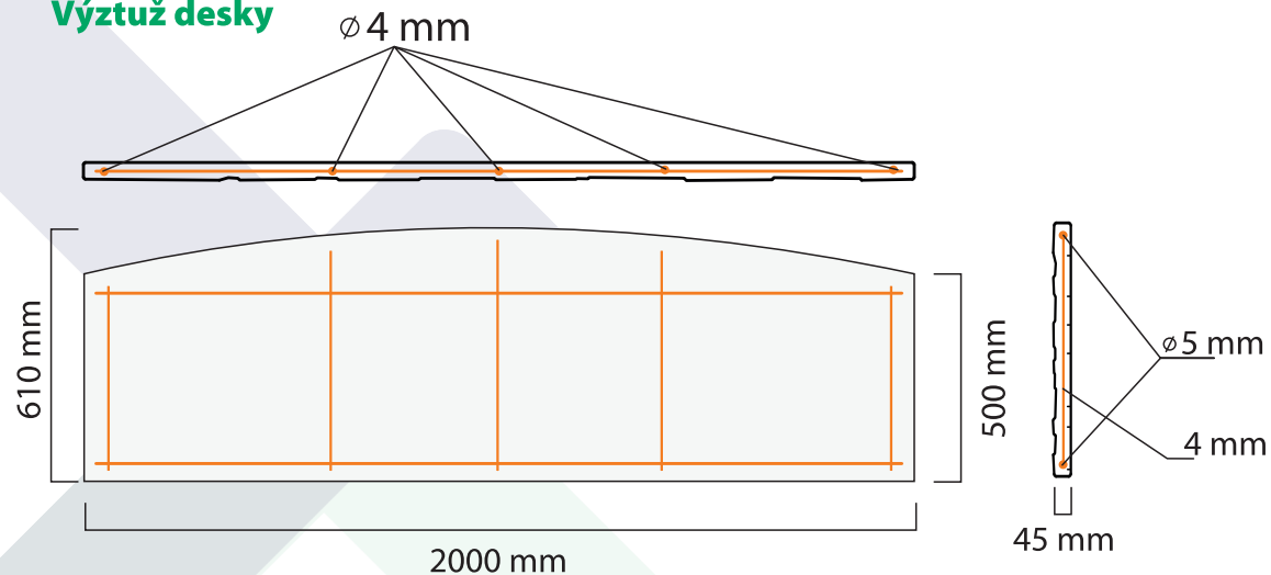
Výztuž desky
